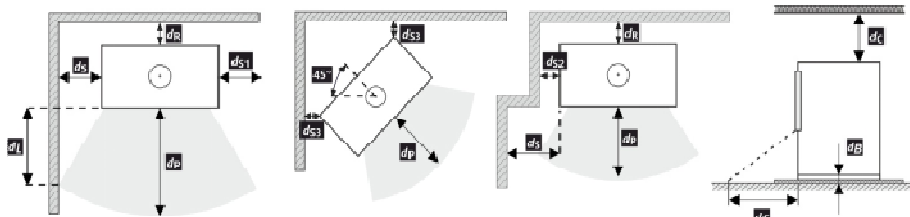
Obrázek 18—náčrtek bezpečných vzdáleností pro umístění spotřebiče typ VSP-9112 a VSP-9112-V
