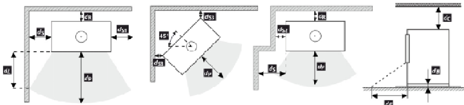
Obrázek 16 – náčrtek bezpečných vzdáleností pro umístění spotřebiče typ VSP-9100, 9100-V a VSP-9103
